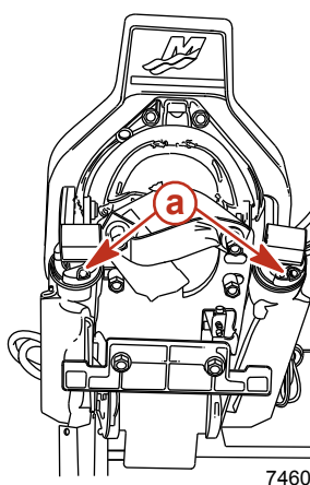
a - Trimmzylinderanoden
