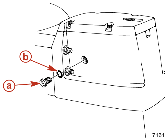
a - Entlüftungsschraube
