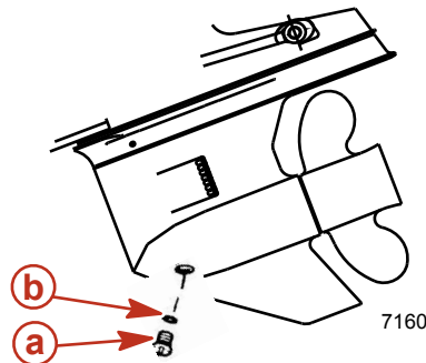
a - Öleinfüll-/ablassschraube
