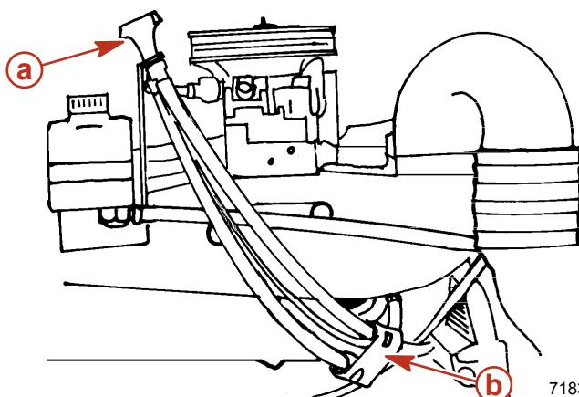
a - Ankergriff
