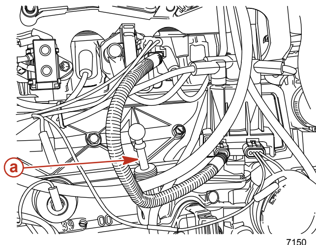
a - Peilstab-Führungsrohr
