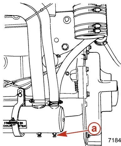
a - Ablassschraube des Wärmetauschers
