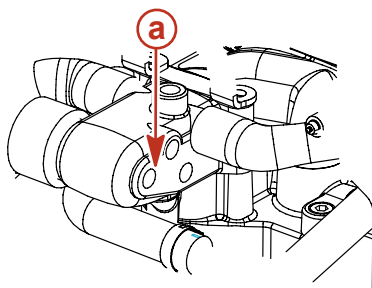
a - Lage des blauen Ablassstopfens
