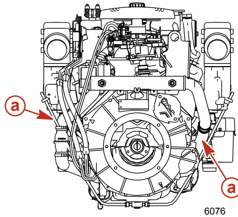
a - Peilstab-Führungsrohr
