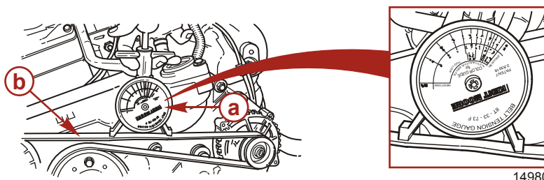
a - Kent Moore© Riemenspannungsmesser
